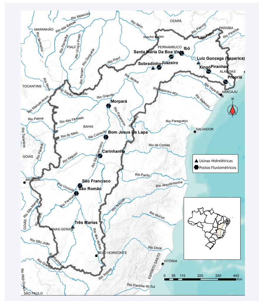
Figura 48. Bacia hidrográfica do rio São Francisco e suas principais UHEs e postos fluviométricos
