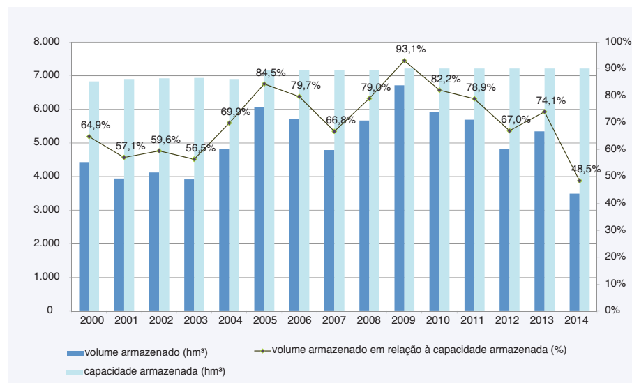
Figura 66. Evolução do percentual de armazenamento de água em reservatórios de UHEs na RH do São Francisco
