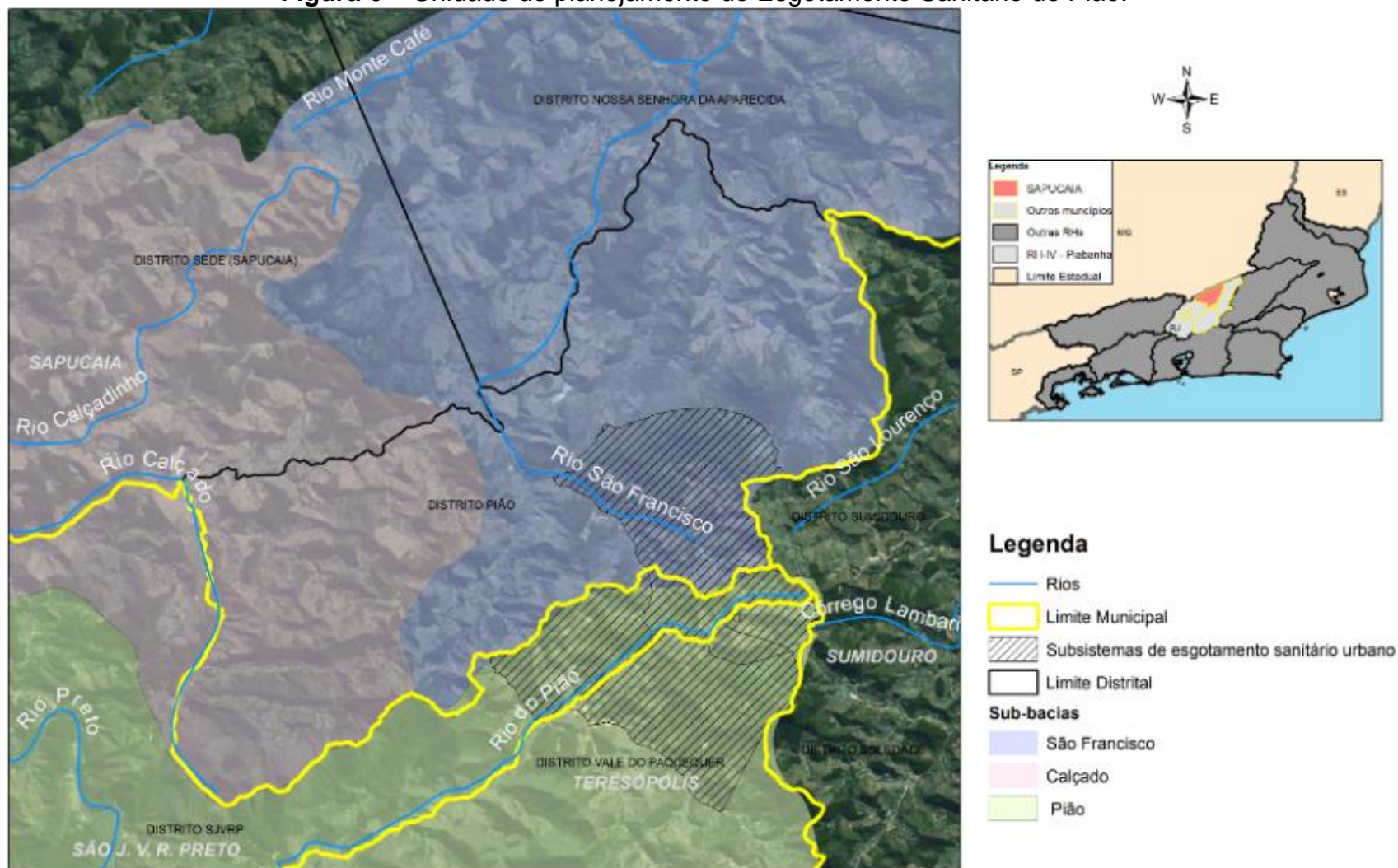
Figura 6 – Unidade de planejamento do Esgotamento Sanitário de Pião.
