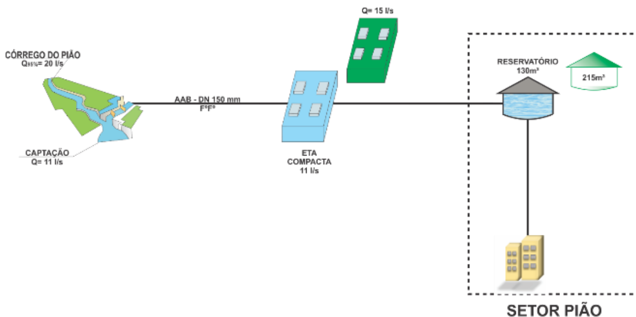
Figura 3 – Esquema do sistema de abastecimento de água proposto para a unidade de planejamento de Pião – metas de curto prazo a serem implementadas até 2019.
