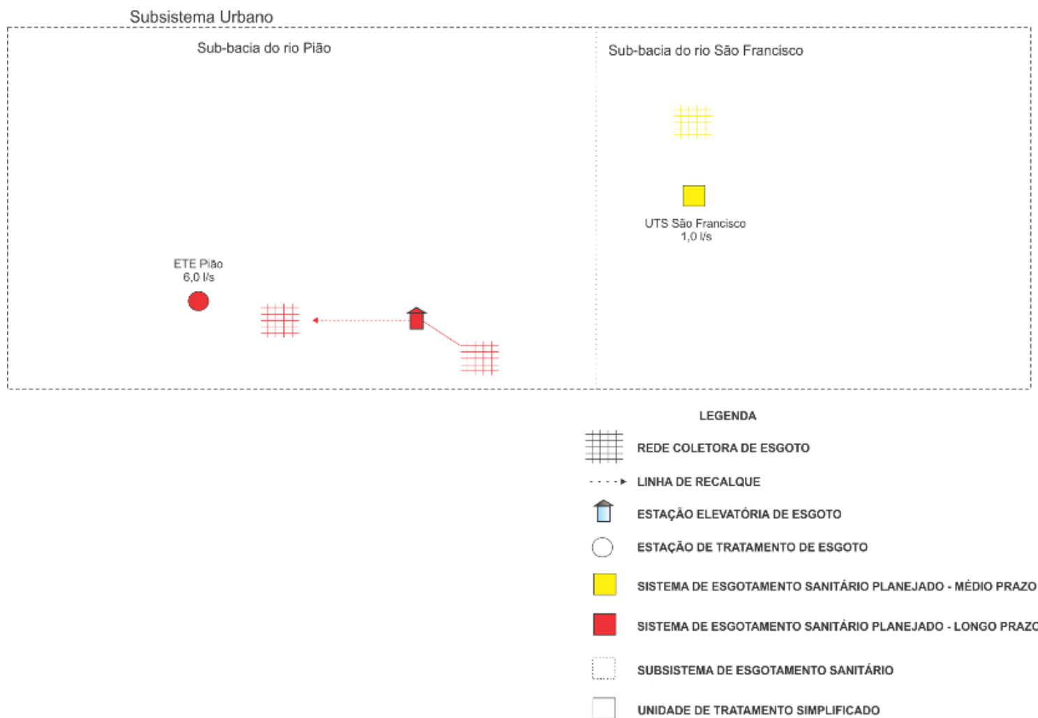
Figura 8 – Esquema com a etapalização da concepção do sistema de esgotamento sanitário urbano de Pião.
