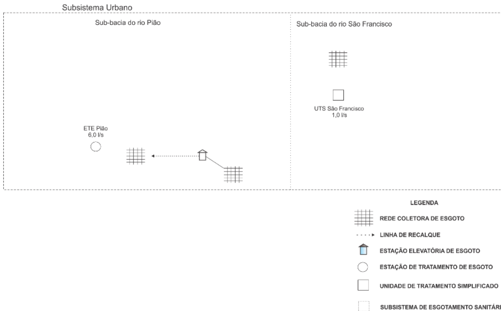
Figura 7 – Esquema com a concepção do sistema de esgotamento sanitário urbano da unidade de planejamento Pião.
