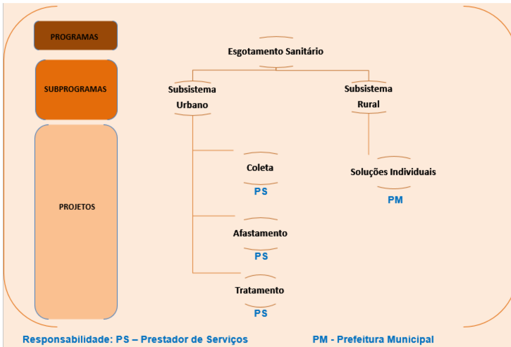
Figura 10 – Fluxograma do programa Esgotamento Sanitário e respectivos subprogramas e projetos.
