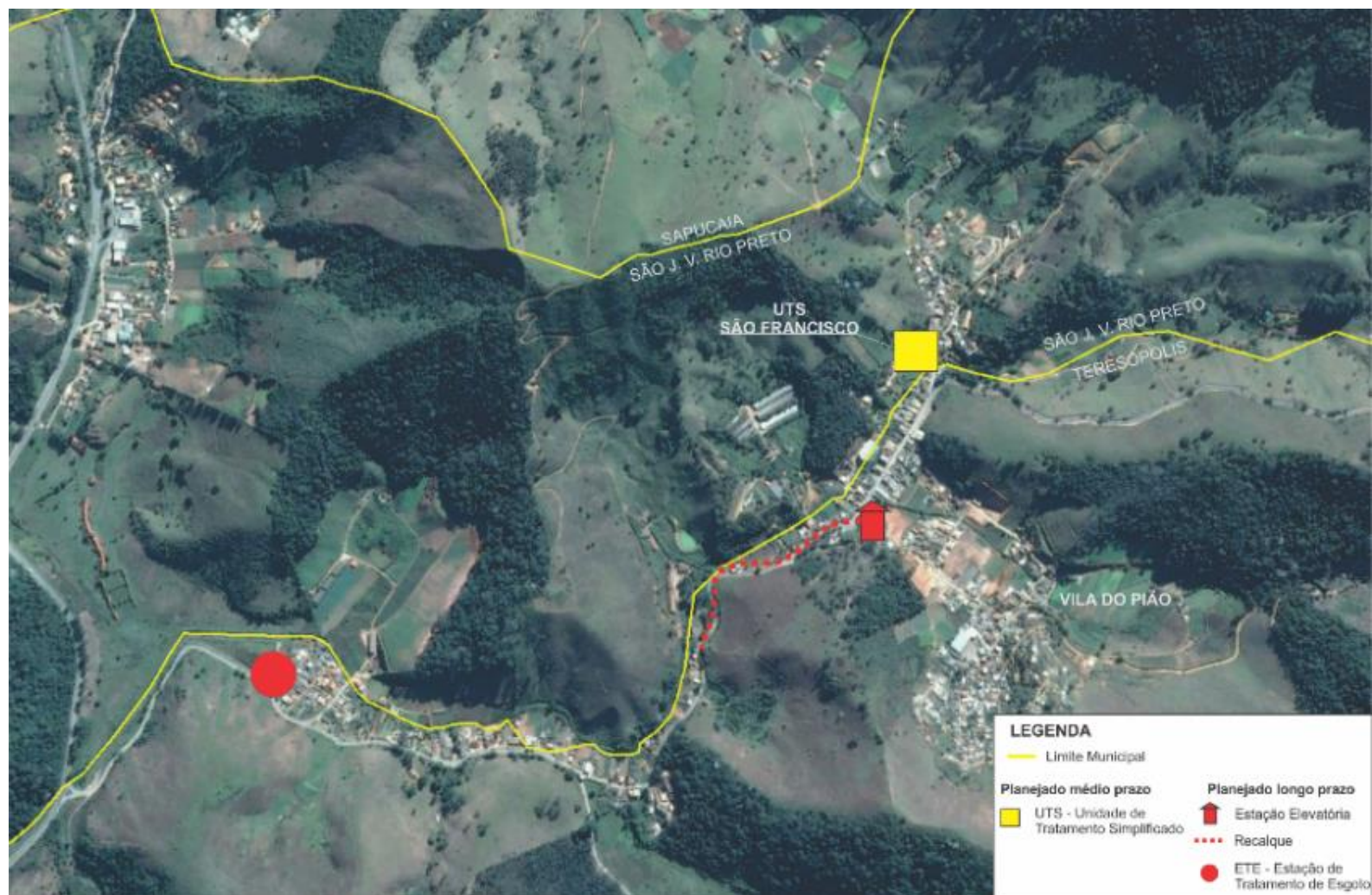
Figura 9 – Mapa a partir de satélite com o sistema de esgotamento sanitário planejado ao longo do Plano.
