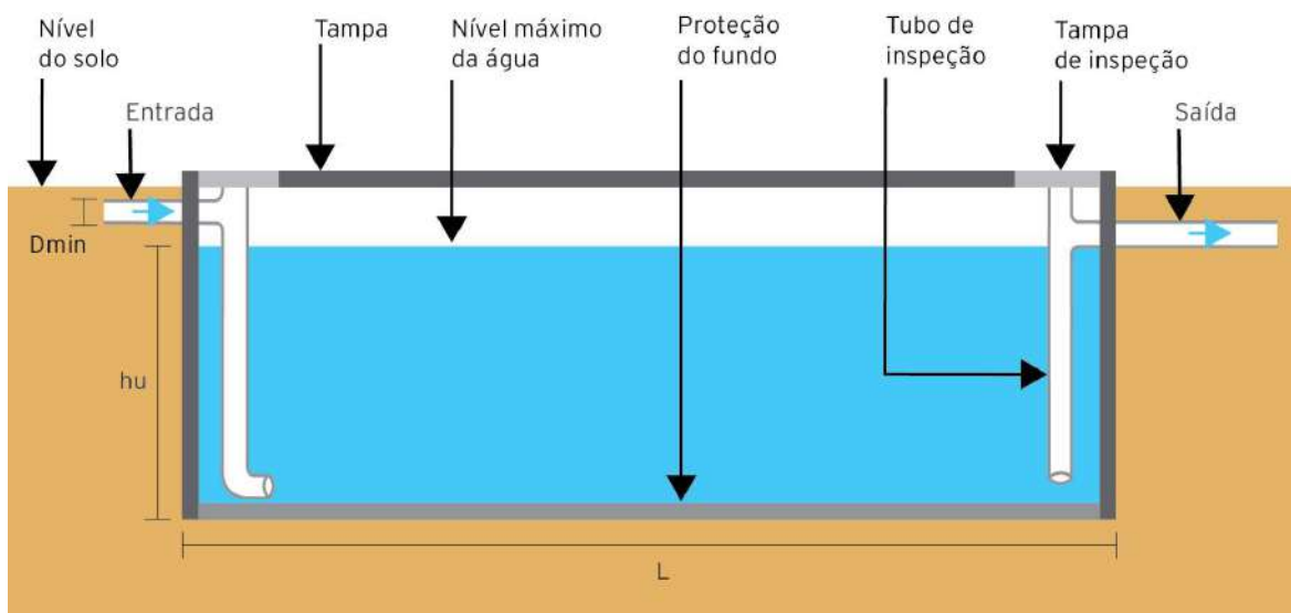
Figura 72 Trincheira de Infiltração sem Preenchimento - Corte Lateral.
