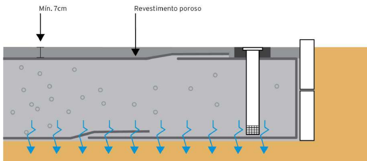
Figura 122 Seção típica de pavimento poroso, com infiltração, acabado. No caso de pavimentos sem infiltração, o fundo e as laterais são revestidos de material impermeável.
