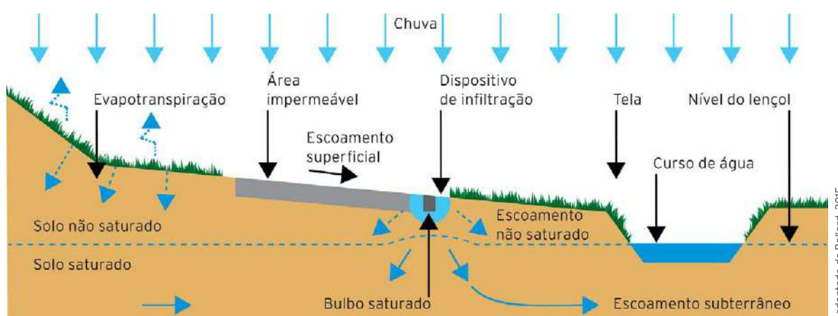
Figura 55 Funcionamento de um sistema de infiltração típico.
