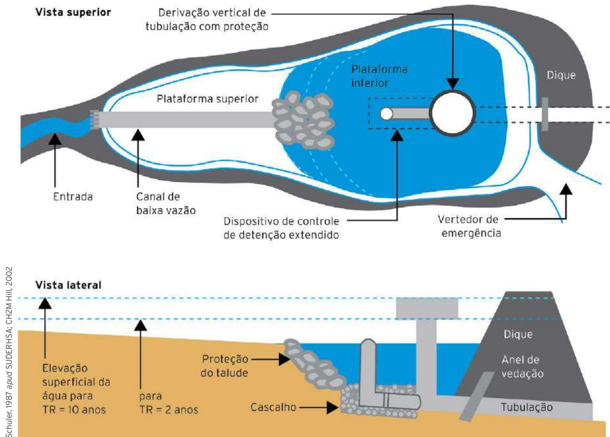
Figura 86 Reservatório de detenção aberto típico.
