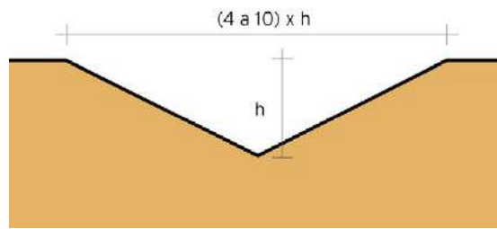
Figura 124 Relações típicas entre largura e altura de valas de infiltração.
