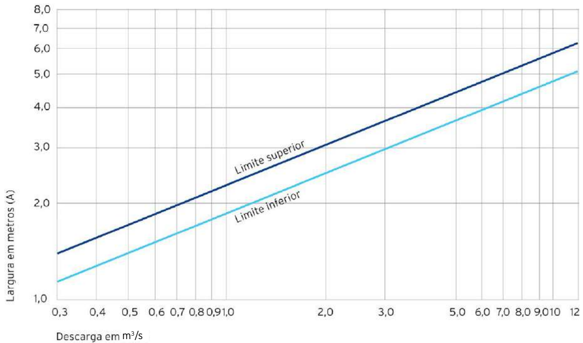
Figura 25 Ábaco de dimensionamento do dissipador por impacto.
